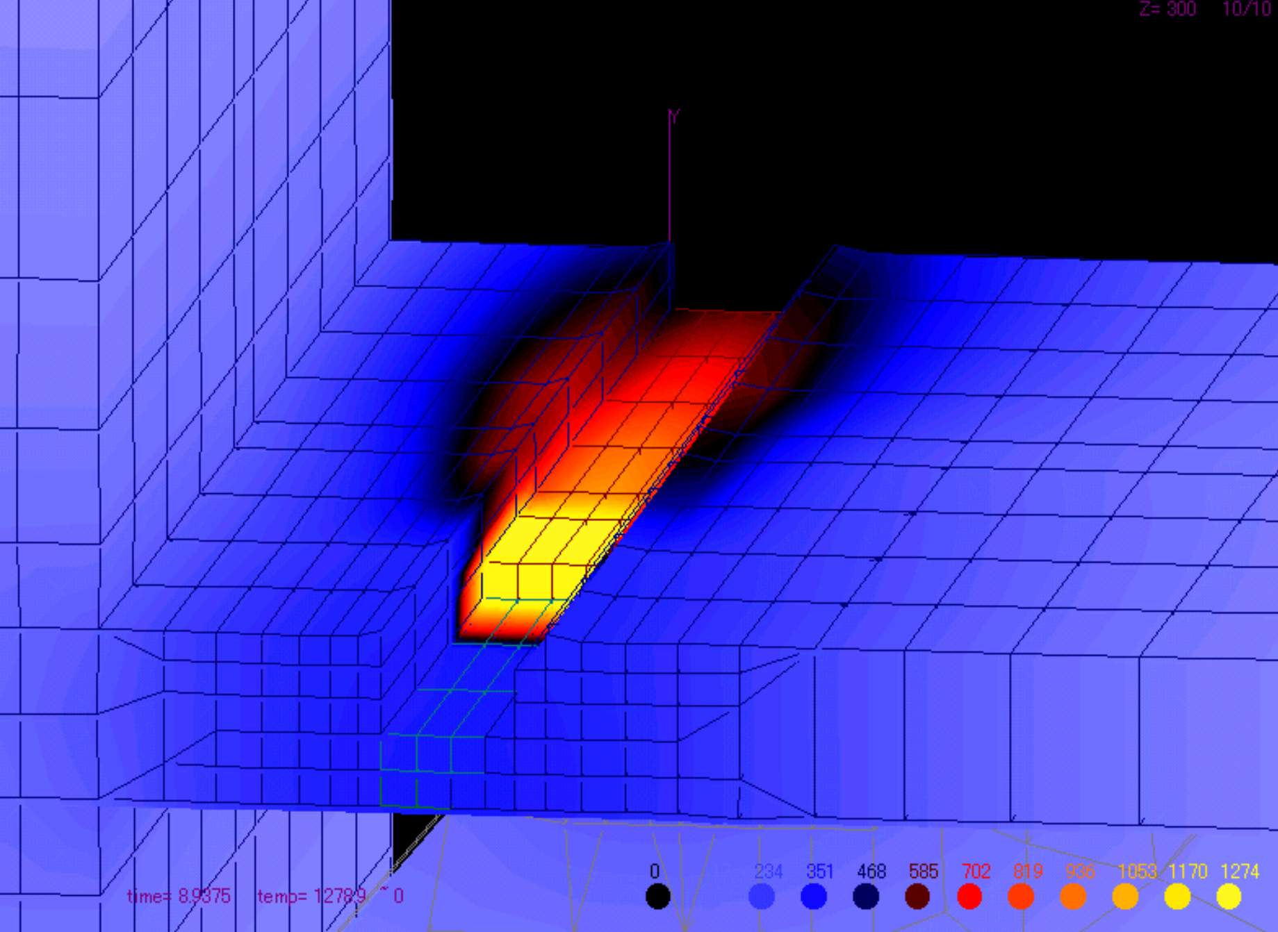
柱—梁接合部3層目溶接中の温度分布
